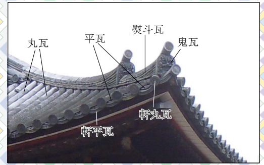
瓦の名称
