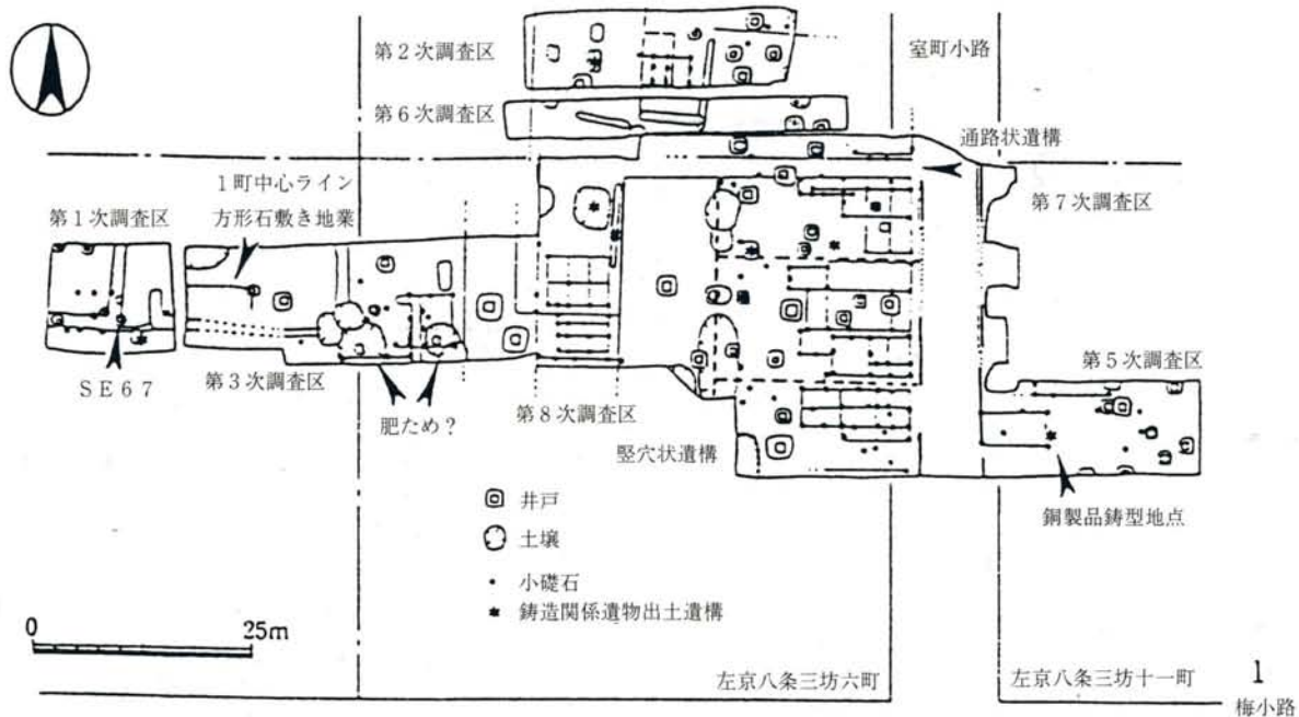
第3図 平安京左京八条三坊六・十一町遺構配置図 (網他1966に加筆)
