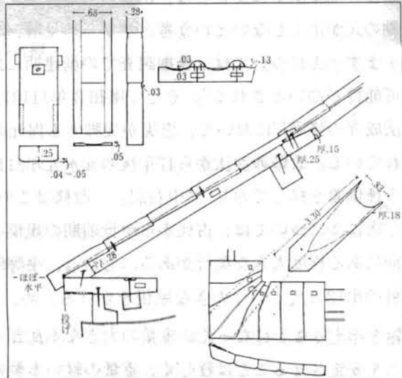
【図⑥】中尊寺金色堂木瓦詳細図
