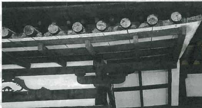
【図⑧】当麻寺曼荼羅堂閼伽棚屋根詳細
