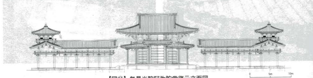
【図11】無量光院阿弥陀堂復元立面図
