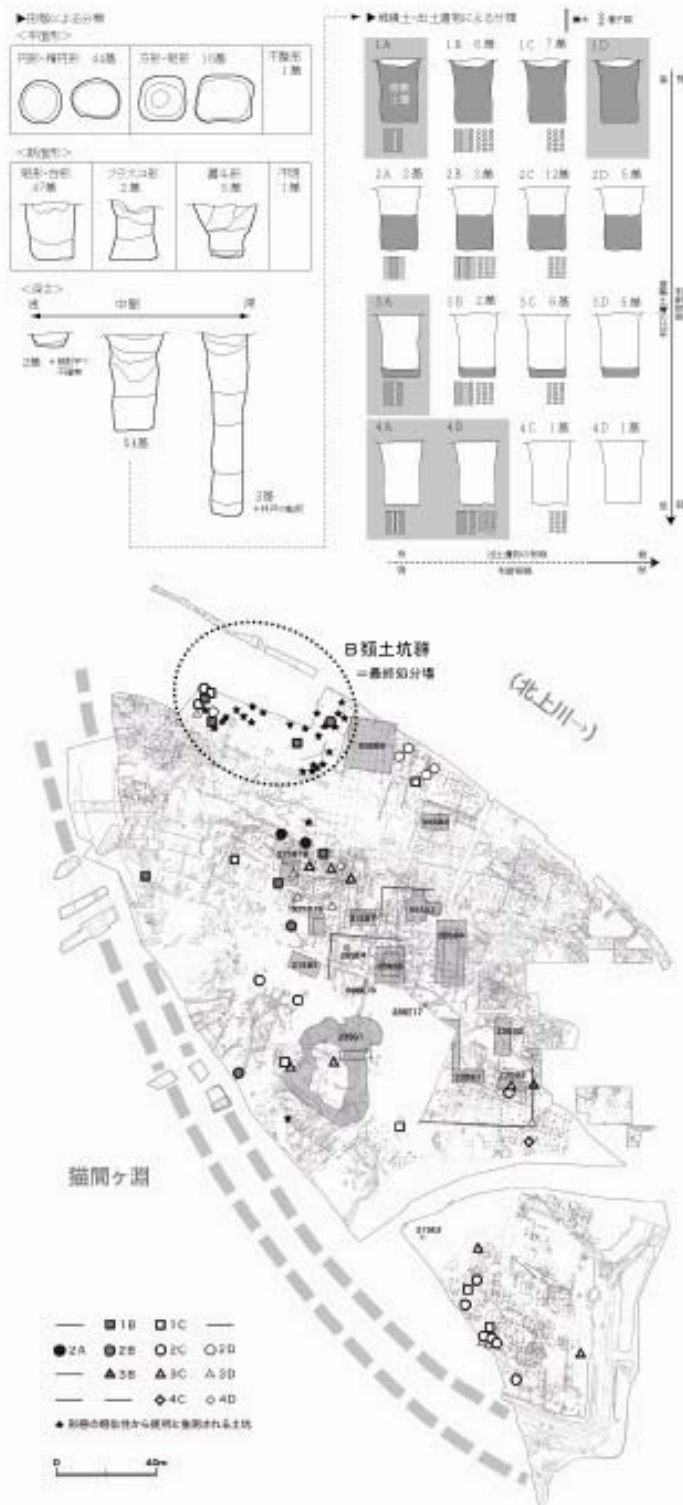
図9 柳之御所遺跡内部地区におけるトイレ状遺構の分類と分布
