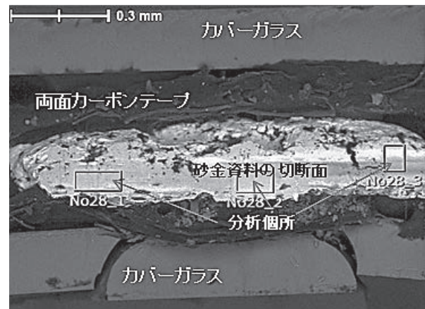
図5. 分析試料のSEM像 (COMP像)
