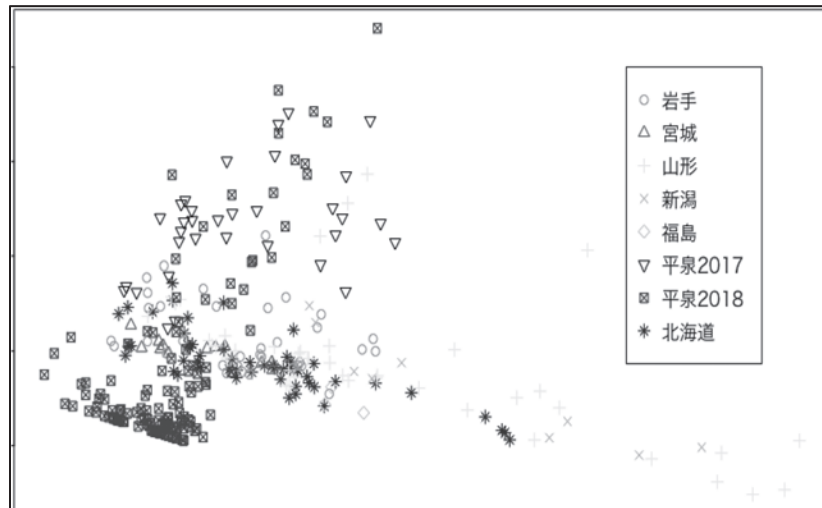
図11. 主成分分析による可視化（横軸：第1主成分、縦軸：第2主成分）
