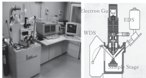
図3. 電子プローブマイクロアナライザー (日本電子製 JXA8900-EPMA 装置)
