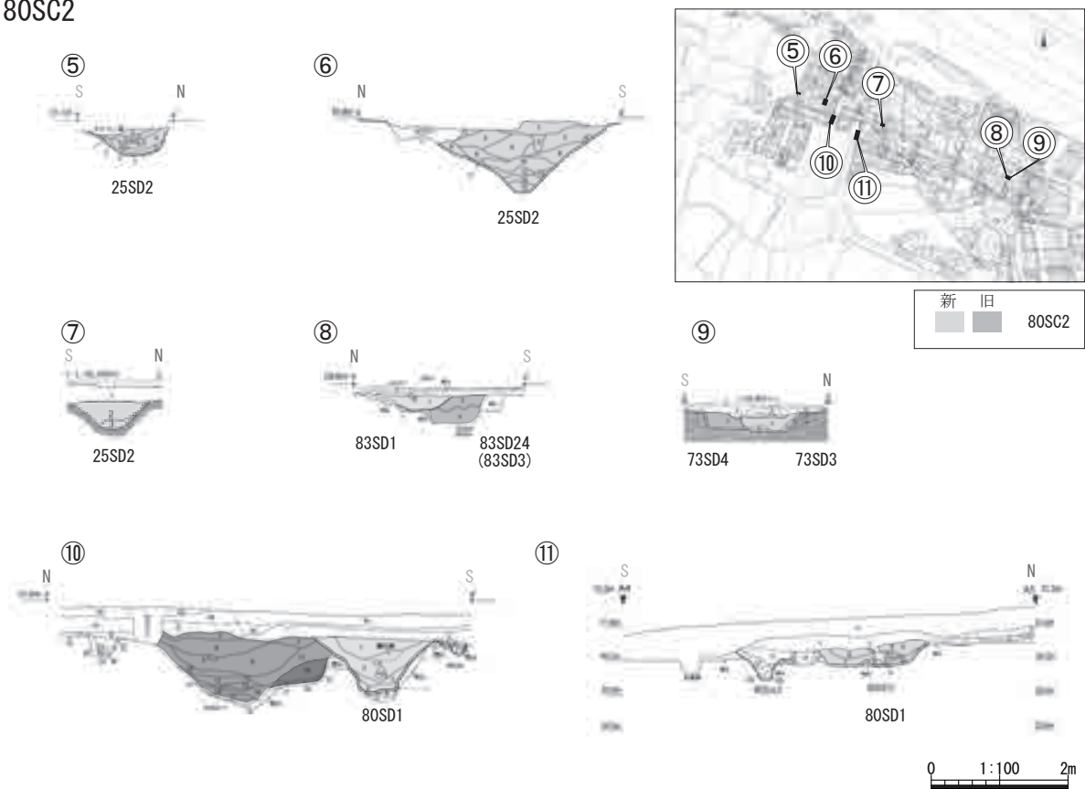
図4 80SC1・80SC2断面集成図
