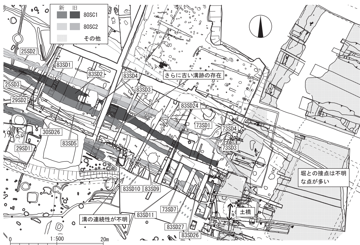
図3 土橋周辺の道路側溝
