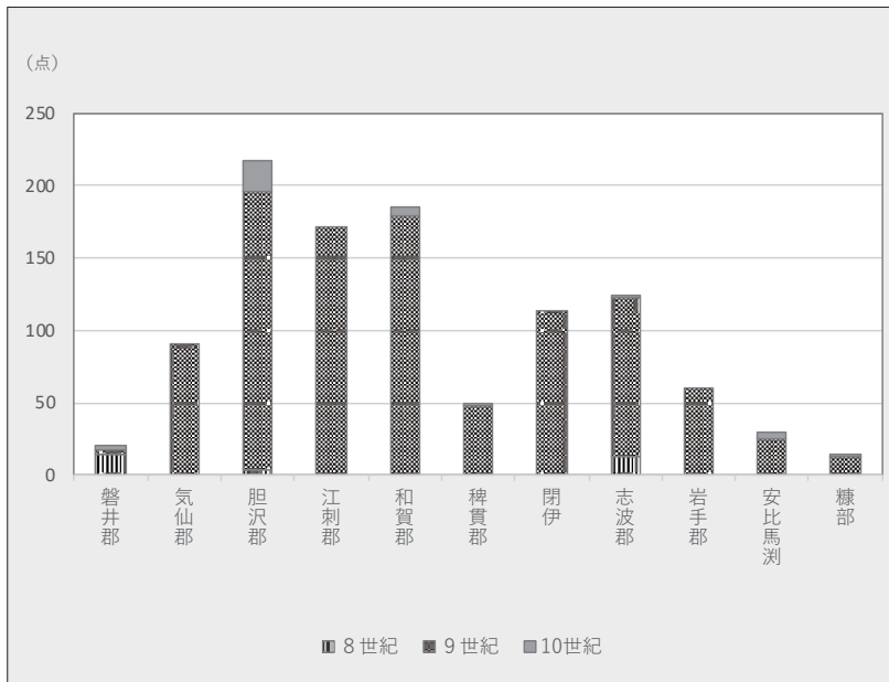
図10 奥六郡域及びその周辺における墨書土器時期別出土点数
