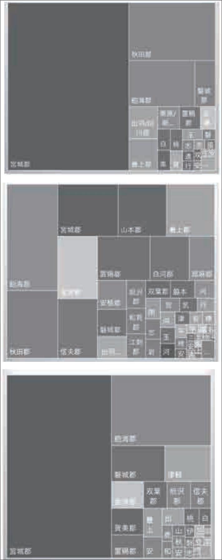
図9 陸奥・出羽における墨書土器出土点数のツリーマップ
