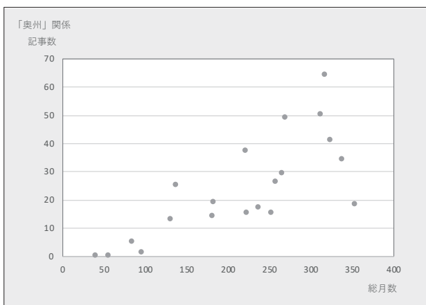
図3 日記総月数と「奥州」関係記事事件数の相関
