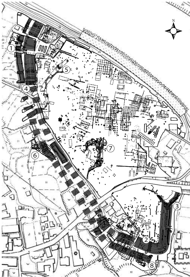
柳之御所遺跡の橋
